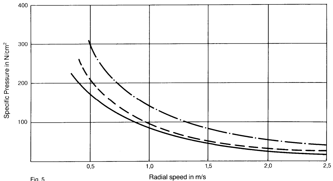
Fig. 5 p · v-diagram Slide bearings
