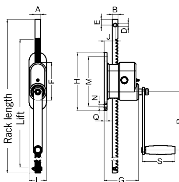
ZWW-L, Capacity 300 - 600 kg
